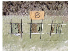
ライニング施工年1987年 19年経過後に外部試験会社による付着強度試験を行う
